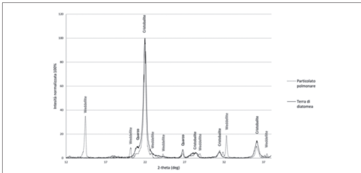
Figura 1 - Diffrattogramma (DRX) del campione commerciale (terra di diatomea-linea continua) in cui si evidenzia il contenuto di cristobalite e piccole quantità di quarzo.
