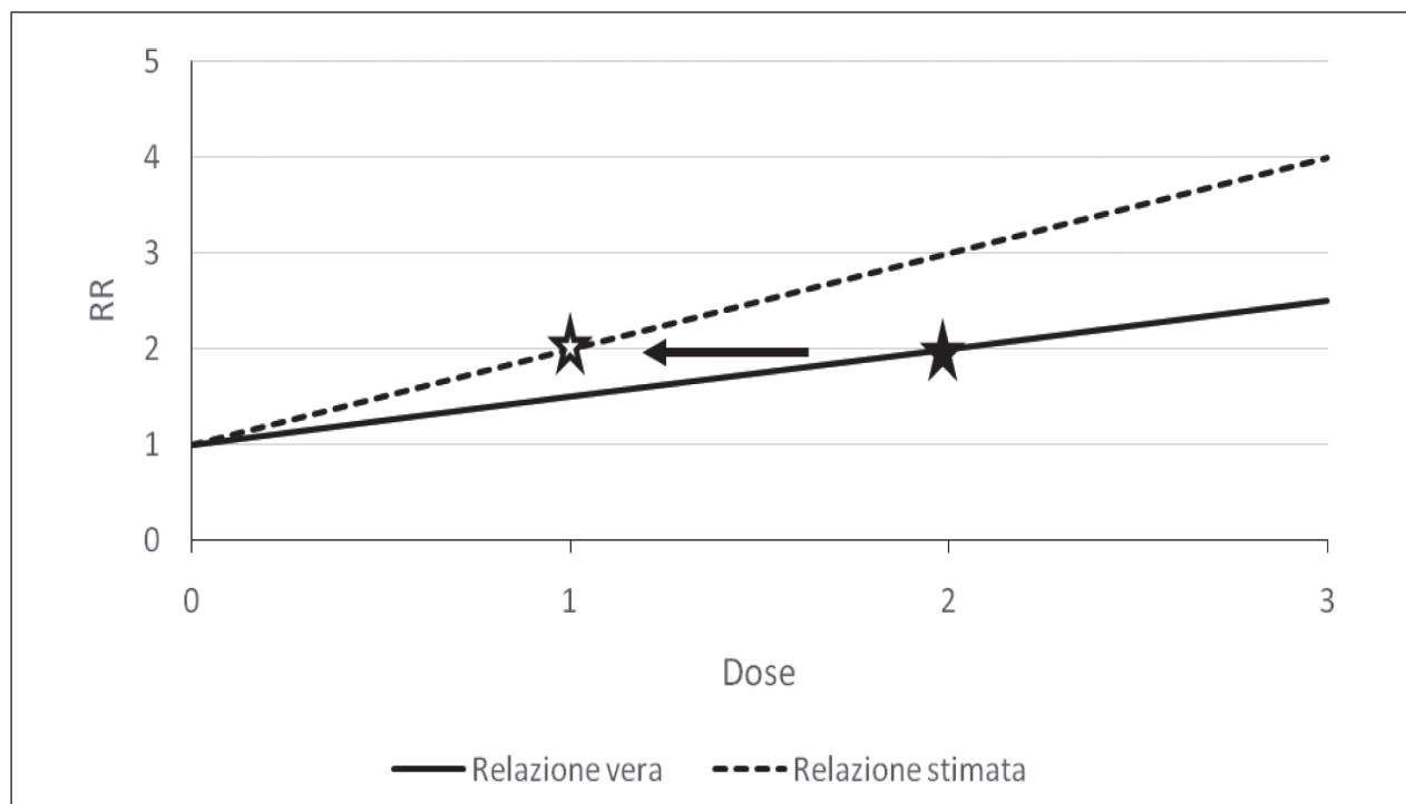
Figura 1 - La vera relazione dose risposta (basata su rischio relativo (RR)=2 a livello 2 della dose (stella piena) è indicata dalla linea continua. A causa della sottostima della dose (freccia), il RR=2 è associato al livello 1 della dose (stella vuota); la corrispondente relazione dose-risposta (sovrastimata) è indicata dalla linea tratteggiata
